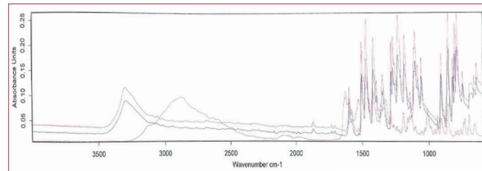
DIE ANALYSE DER INHALTSSTOFFE in einem „Spektrum“ dargestellt.
