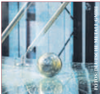
links: Vordächer müssen so konzipiert und befestigt sein, dass sie auch schwere Schneelasten tragen. rechts: Echtglas-Vordächer im Test.
