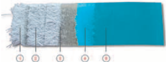
1-3: Glasfasermatten getränkt mit Harz, 4: Vorversiegelung, 5: Endversiegelung in allen RAL-Farben.
