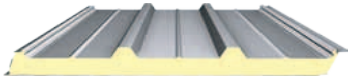
METALLDACHPLATTE mit PU-Kern, wie sie von KANO für die Dachsanierung verwendet wird.
